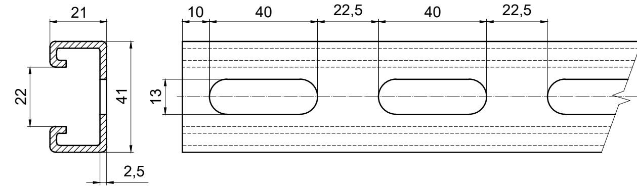
ST41x21x2,5mm
